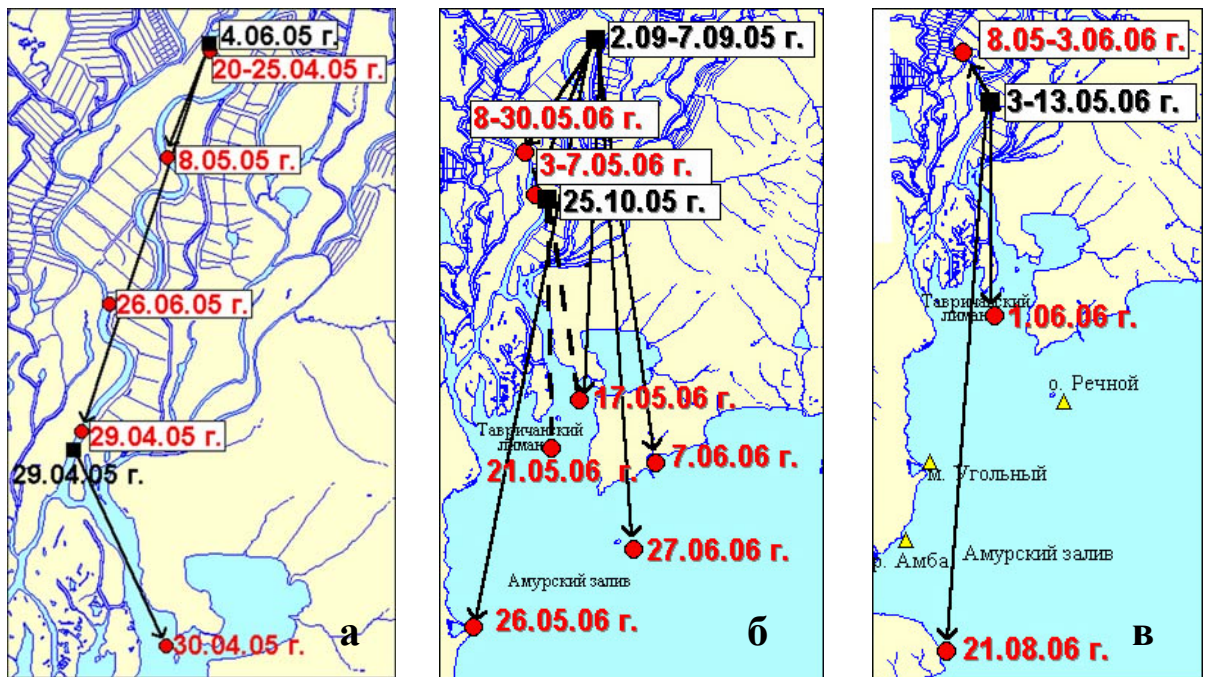
Рис. 2. Перемещения японского мохнаторукого краба в низовьях р. Раздольной в весенне-летний период 2005 и 2006 гг.: квадрат – место выпуска меченых крабов, круг и треугольник – места поимки крабов; черные цифры – даты выпуска, красные цифры – дата поимки. Масштаб: 1 см – 1600 м (а), 2550 м (б) и 2900 м (в)
