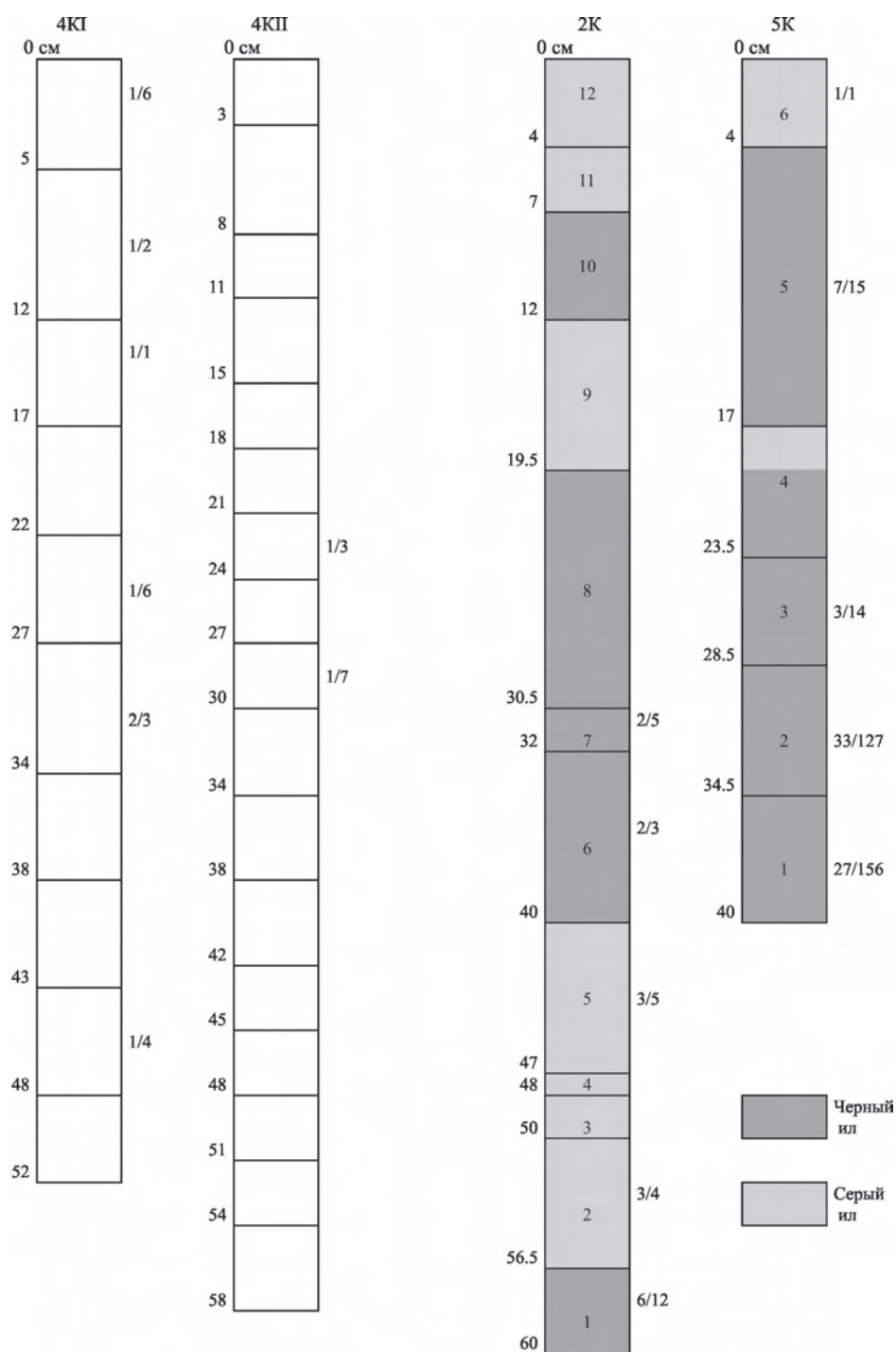
Рис. 3.3. Характер распределения видов и створок остракод в колонках осадков гавани в б. Гайдамак. Числа слева от колонок – глубина, в см; числа справа от колонок: в числителе – количество видов, в знаменателе – количество створок; цифры внутри колонок – номера интервалов
