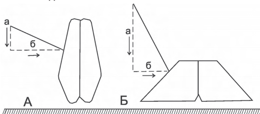
Рис. 2.2. Разложение силы давления потока на раковины остракод с крутой (А) и покатой (Б) поверхностью верхней части раковины: а – придавливающая сила; б – сносящая сила (объяснения см. в тексте)
