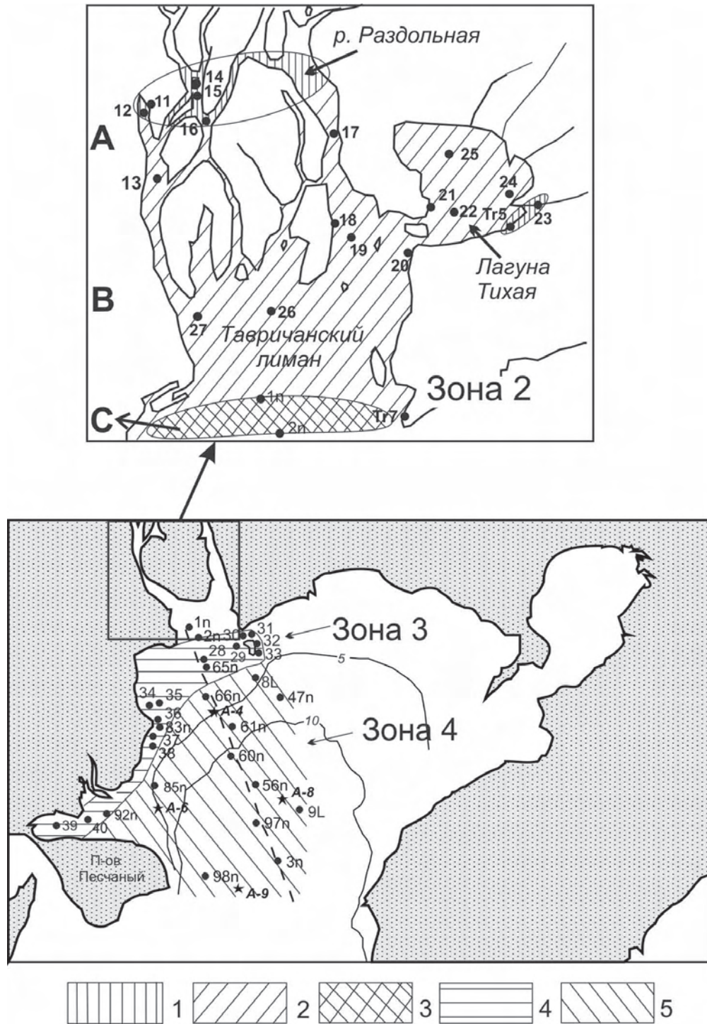
Рис. 6.3. Зоны и подзоны распределения комплексов остракод в районе эстуария р. Раздольная в зависимости от солености воды: 1 – подзона 2А, 2 – подзона 2В, 3 – подзона 2С, 4 – зона 3, 5 – зона 4
