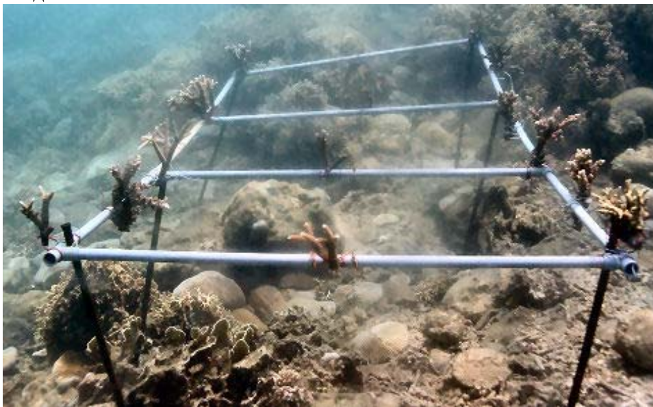
Рис. 74. Экспериментальная установка для выращивания фрагментов кораллов
