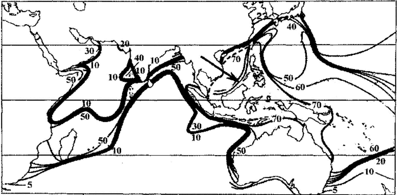
Рис. 16. Карта-схема изолиний родового разнообразия рифообразующих склерактиний в различных регионах Индопацифики (частично по: Veron, 1995). Пунктиром обозначена новая граница изолинии распространения 70 родов, стрелкой - прежняя ее граница.
